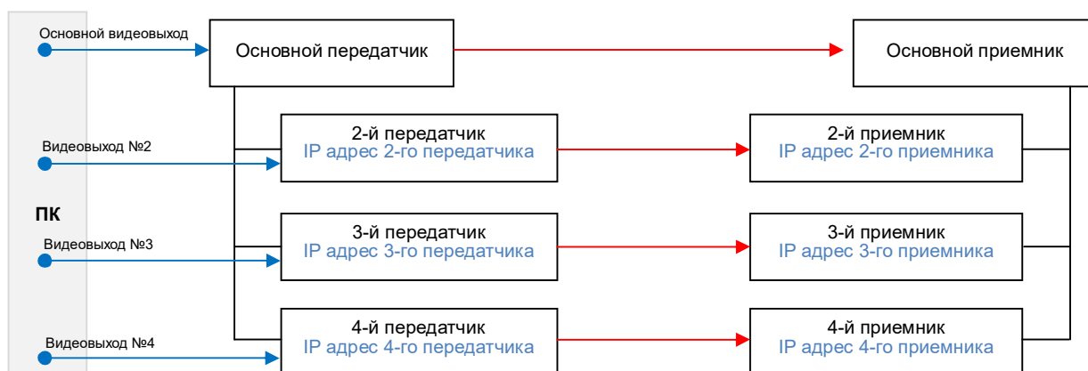
Схема подключения основных и связанных передатчиков и приемников
